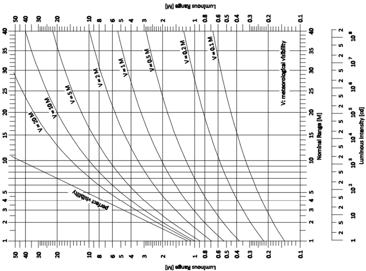
Fig. 2-2 Tabela de Alcance Nominal e Diagrama de Alcances Luminosos – arco diurno . O diagrama tem como base uma iluminância de E_r = 1 \cdot 10^{-3} lx . (Fonte: AISM/IALA, R0202 (E200-2)).
